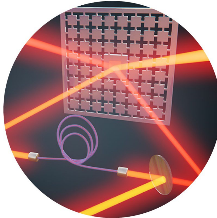
Neue Technik für die Laserkühlung von Membranen
